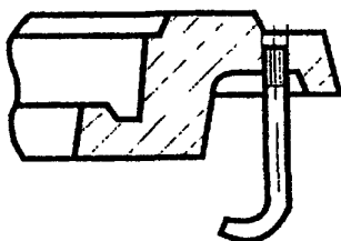
Рисунок А.4 — Усиленная заделка корпуса люка
