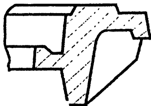
Рисунок А.4 — Усиленная заделка корпуса люка
